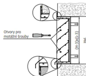
Obr. 1: Detaily žaluzie
